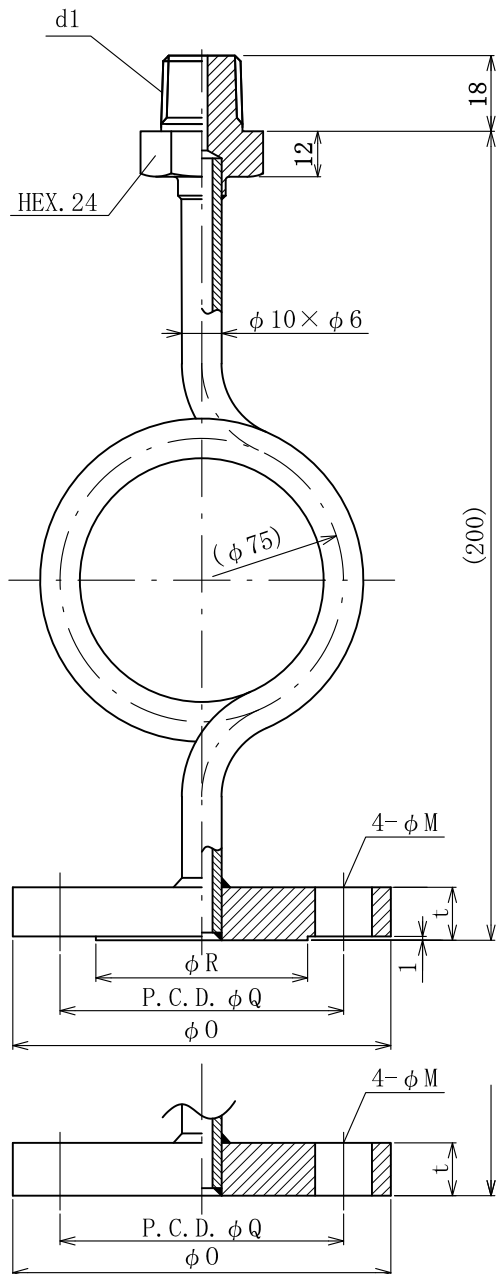
取合フランジ FLANGE CONNECTION 【JIS B2220-2012】
