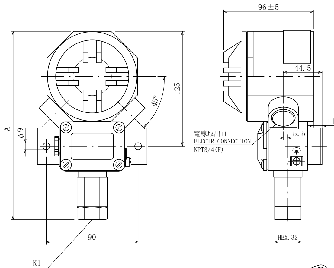
プロセス接続口/PROCESS CONNECTION
