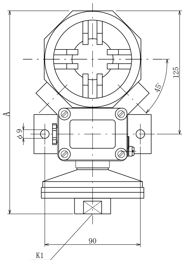
プロセス接続口/PROCESS CONNECTION
