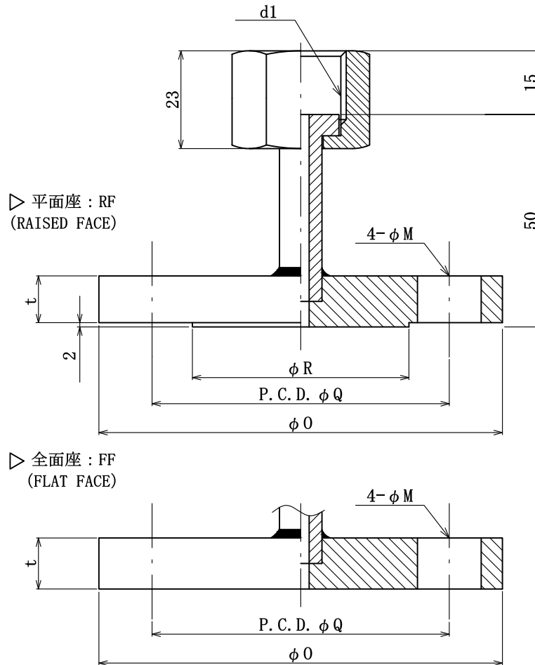
取合フランジ FLANGE CONNECTION 【JPI-7S-15-2011】
