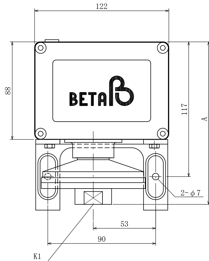
プロセス接続口/PROCESS CONNECTION
