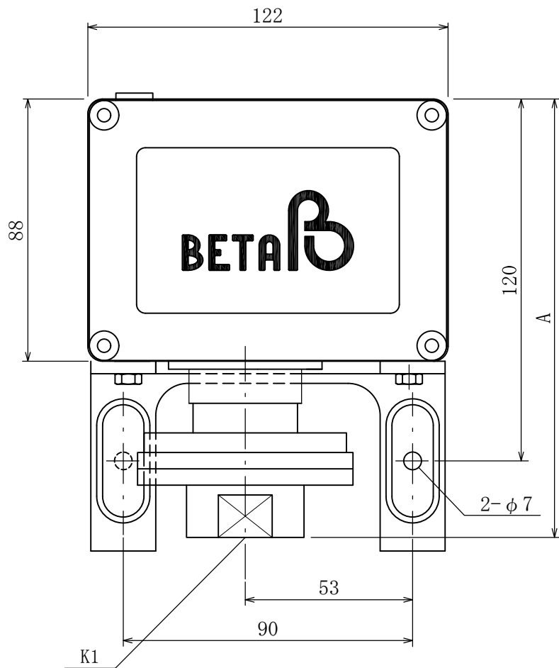
プロセス接続口/PROCESS CONNECTION
