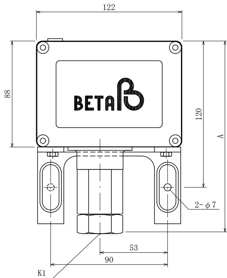
プロセス接続口/PROCESS CONNECTION
