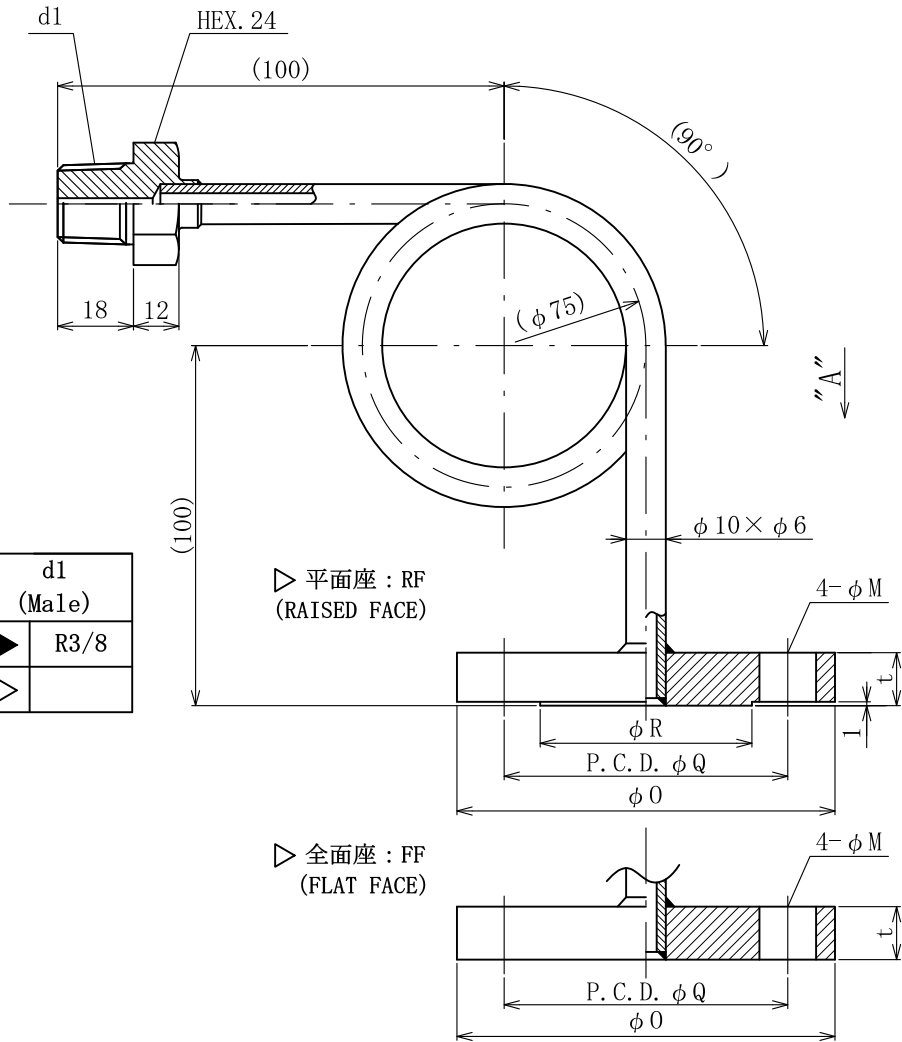
取合フランジ FLANGE CONNECTION 【JIS B2220-2012】
