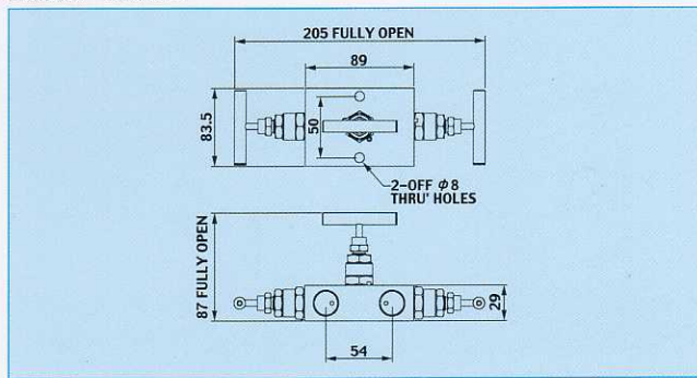
MODEL Q3 3バルブマニホールド Rated 40MPa
