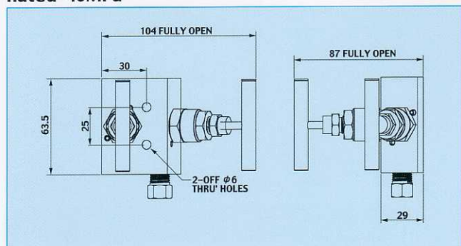
MODEL L2 2バルブ(オス・メス)マニホールド Rated 40MPa
