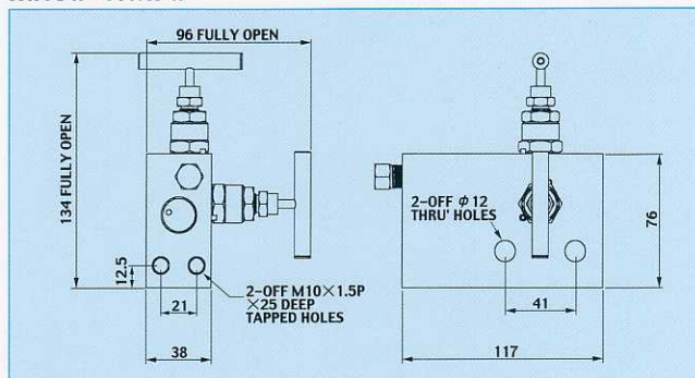
MODEL O2 平型バルブマニフォールド Rated 40MPa
