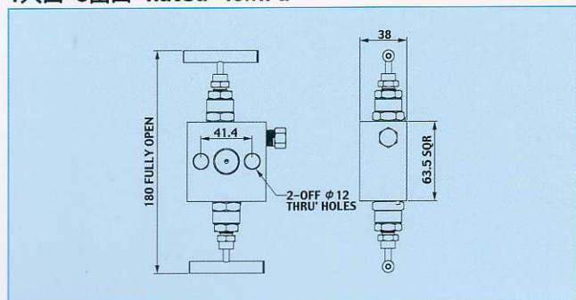
MODEL M2 計器用マルチプラグ 1入口・3出口 Rated 40MPa
