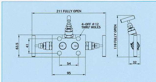
MODEL Q3 3バルブマニホールド Rated 40MPa
