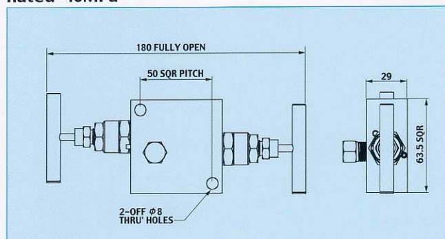
MODEL K2 アングル2型バルブマニフォールド Rated 40MPa
