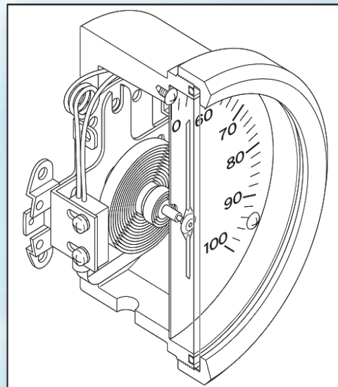
温度計 内部構造図
